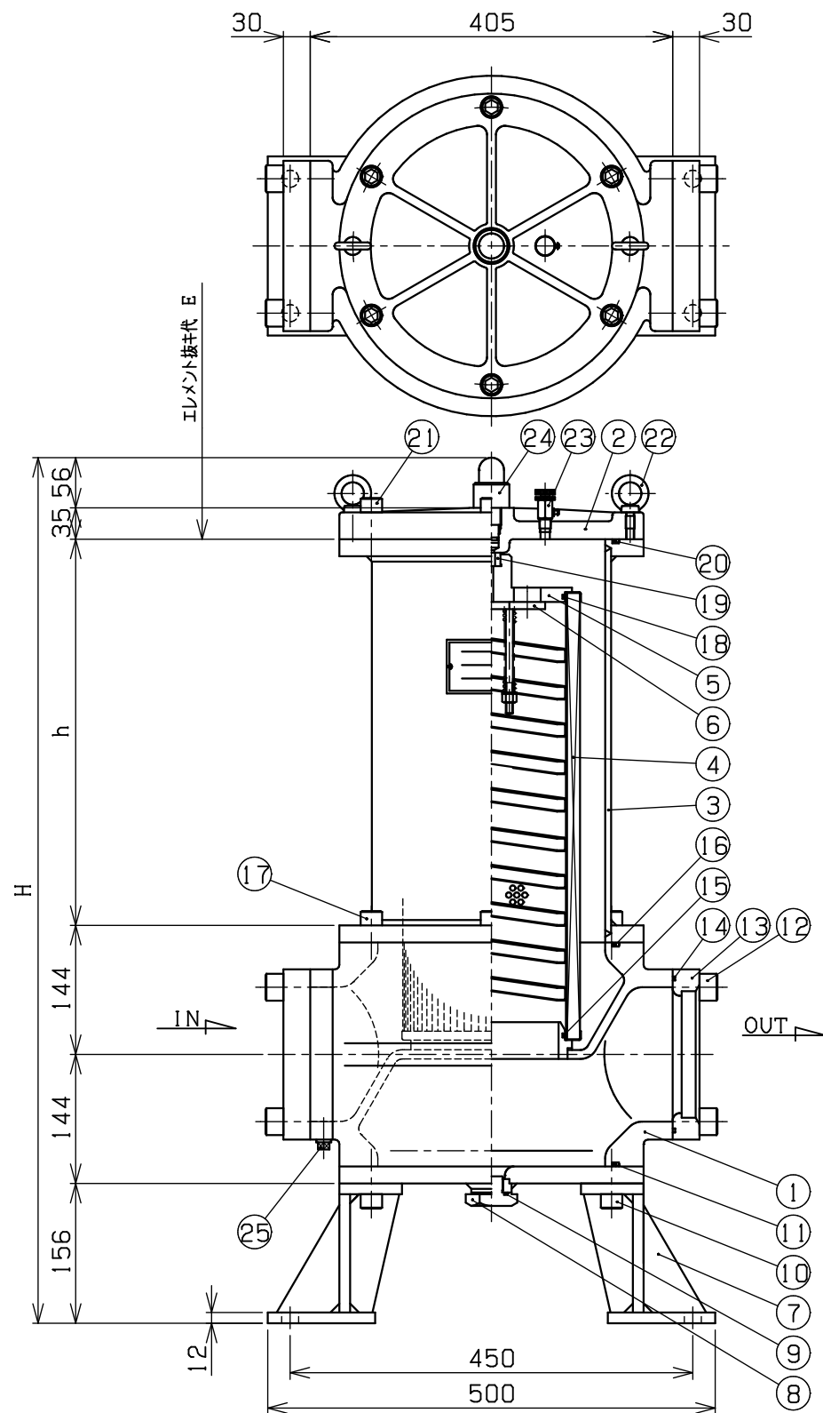
【寸法表（目視形検知器）】
